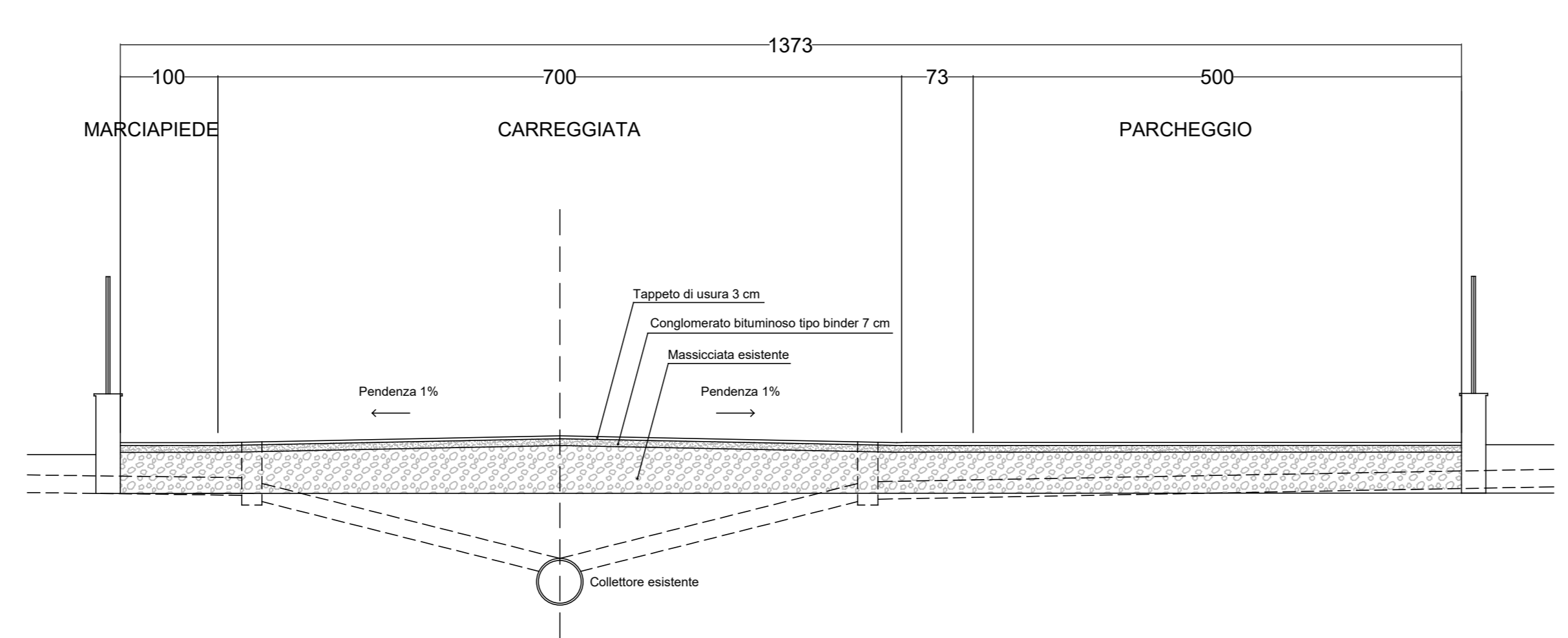
Sezione tipo - BB 1:50
