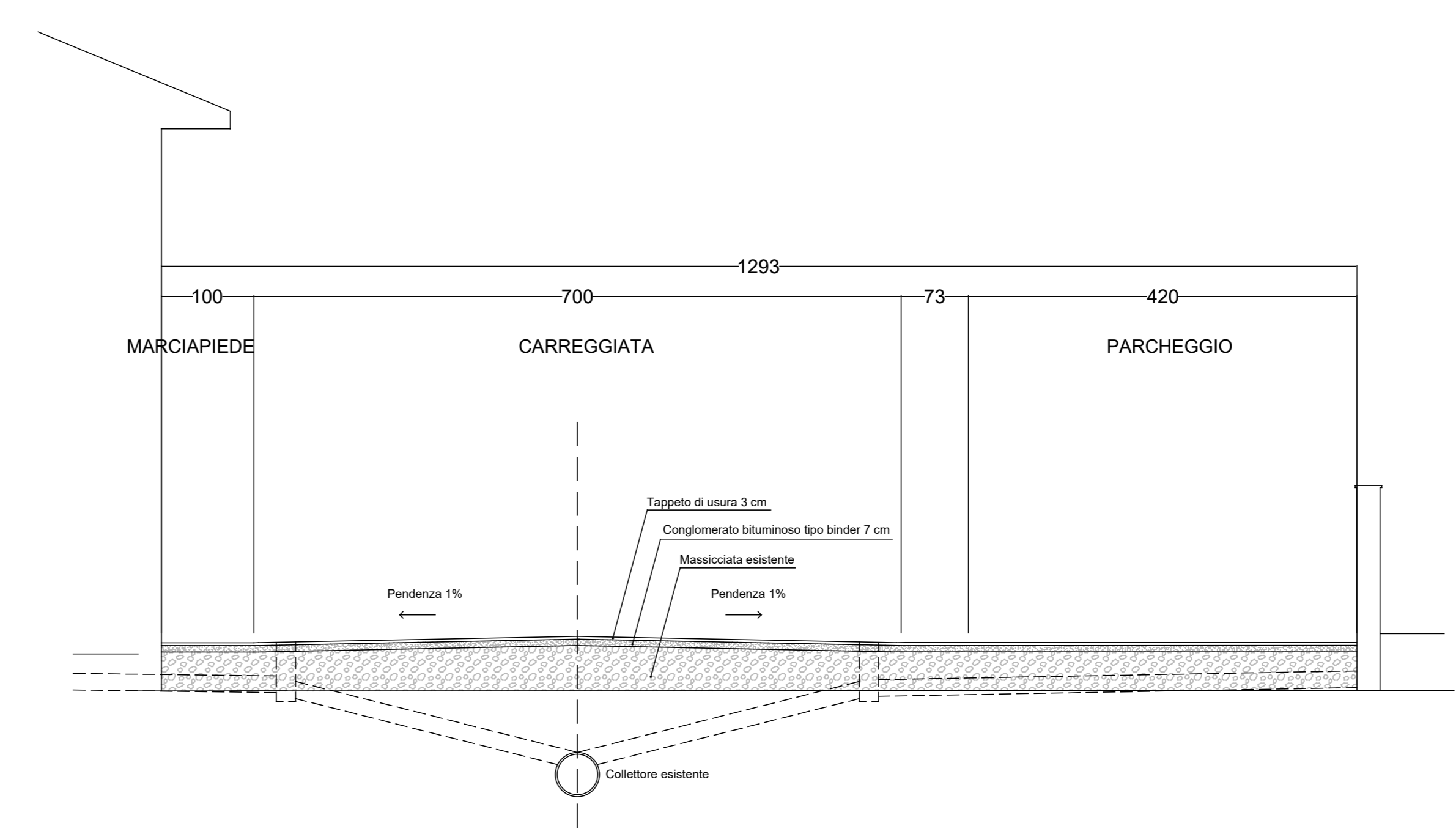
Sezione tipo - CC 1:50
