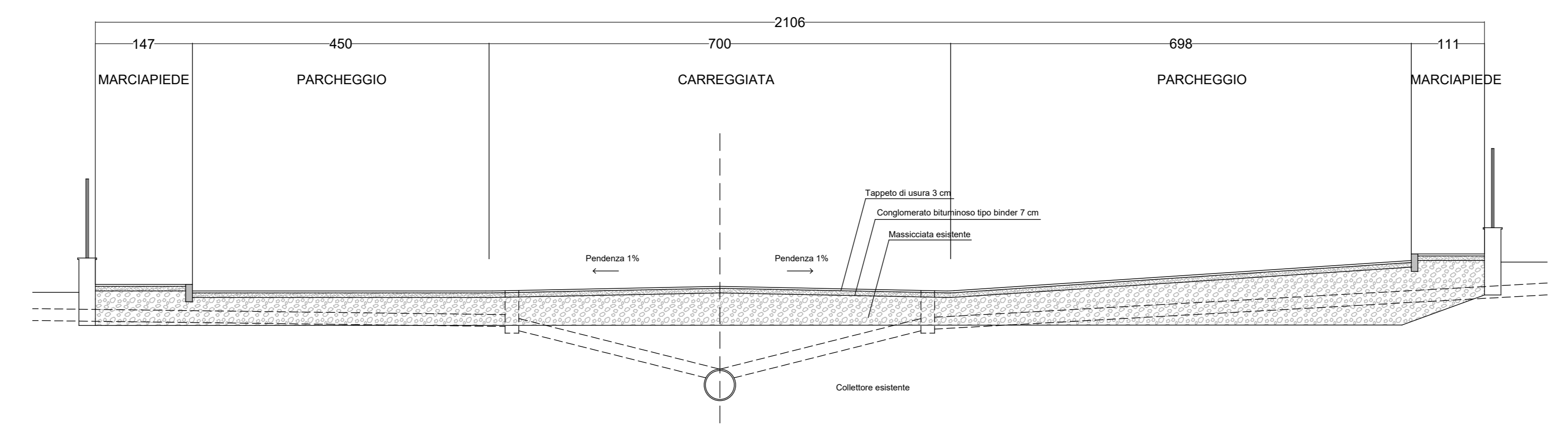
Sezione tipo - AA 1:50
